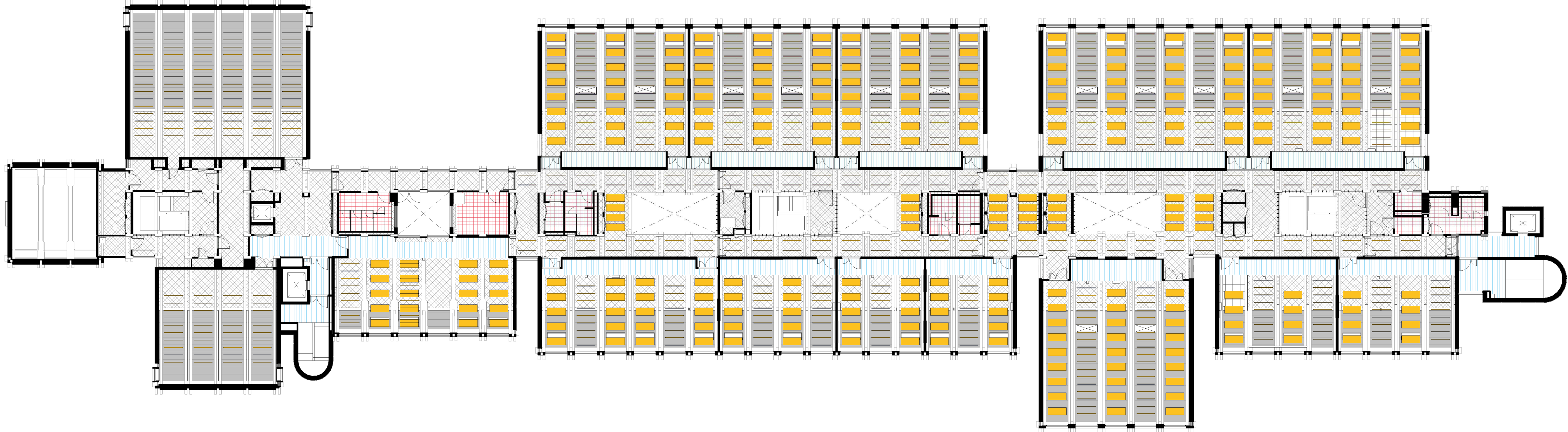
3 13300-Level 2 Plan 1 : 200
