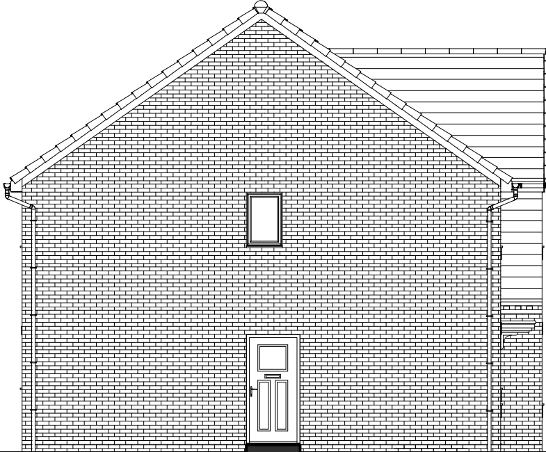
L.H. SIDE
