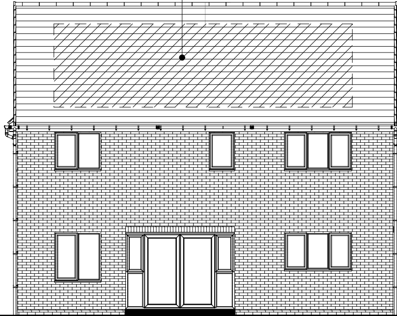
L.H. SIDE
