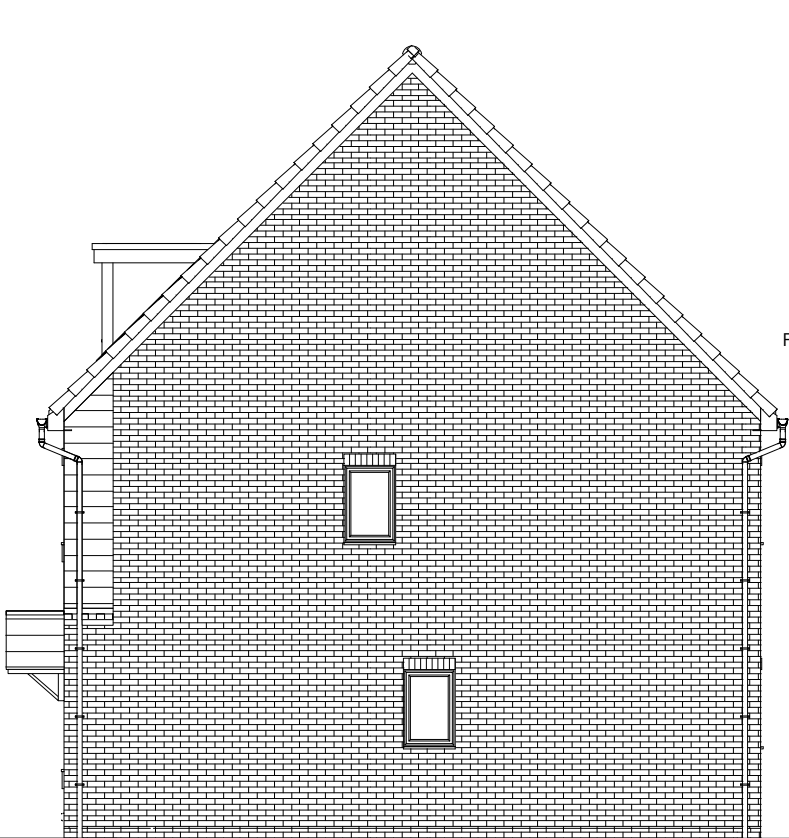
L.H. SIDE
