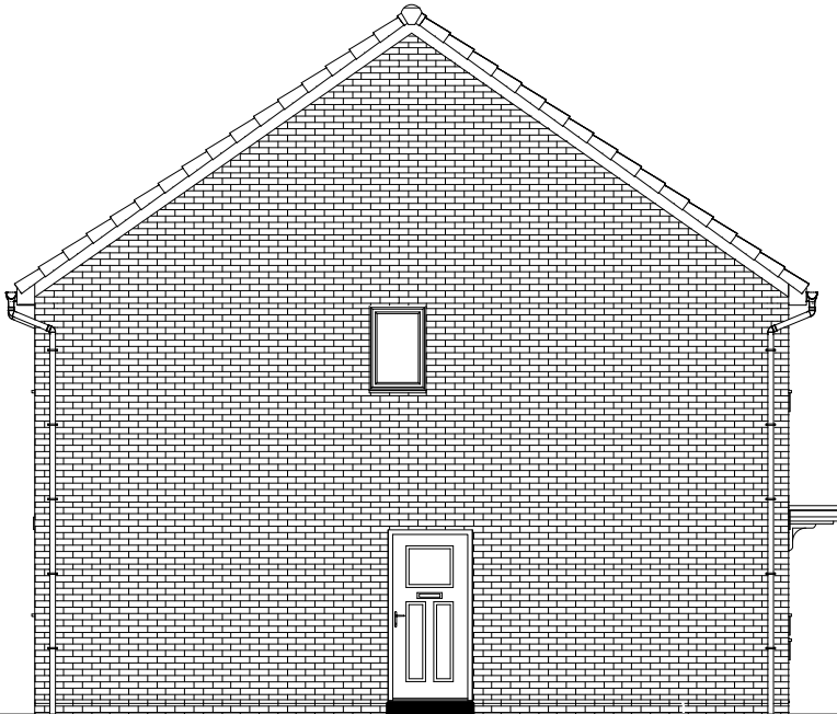
L.H. SIDE
