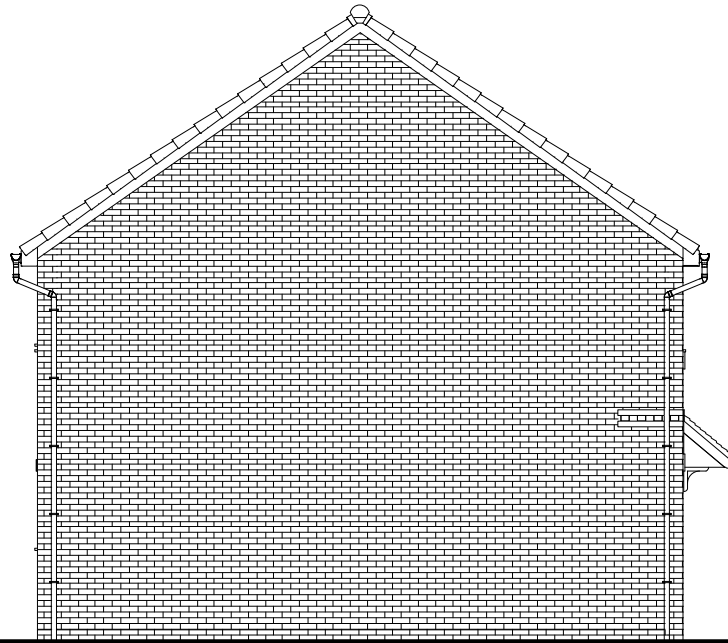
R.H. SIDE
