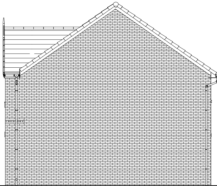
L.H. SIDE
