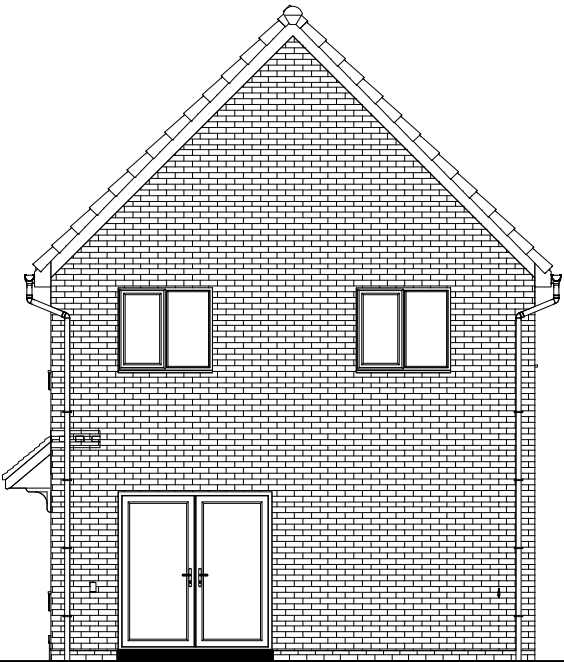
L.H. SIDE
