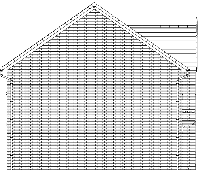
R.H. SIDE
