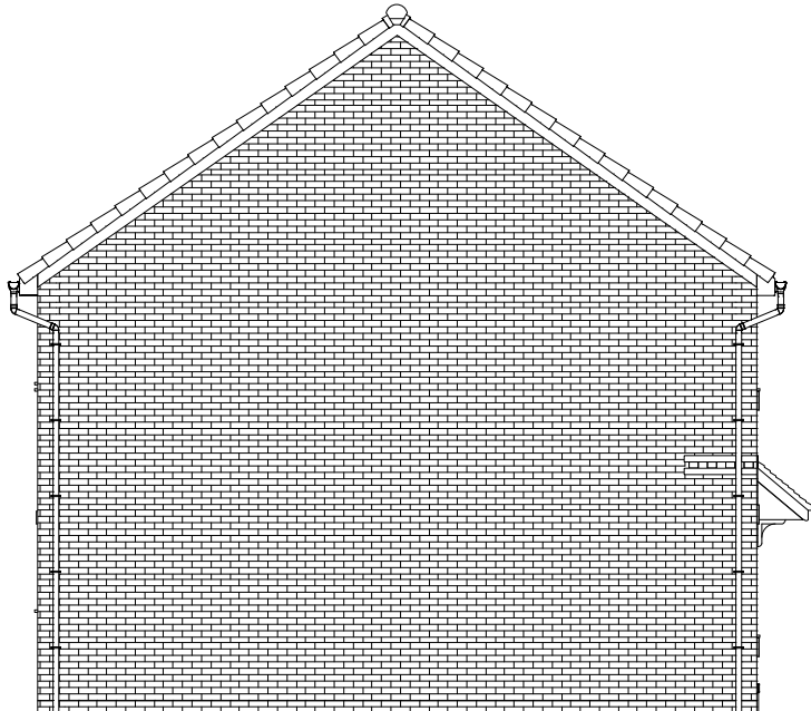
L.H. SIDE
