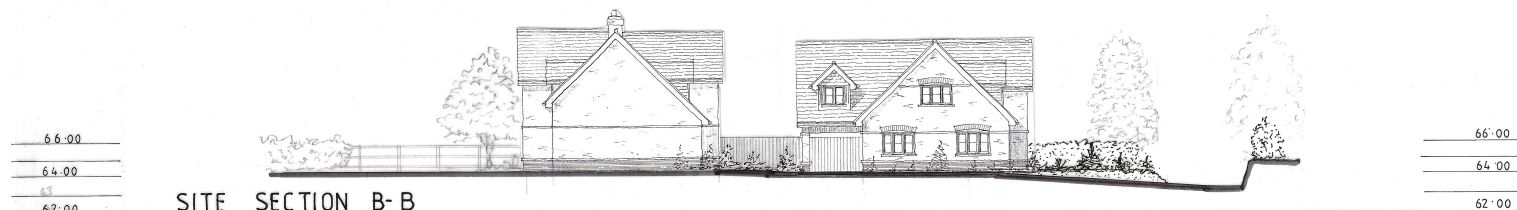
SITE SECTION B-B
