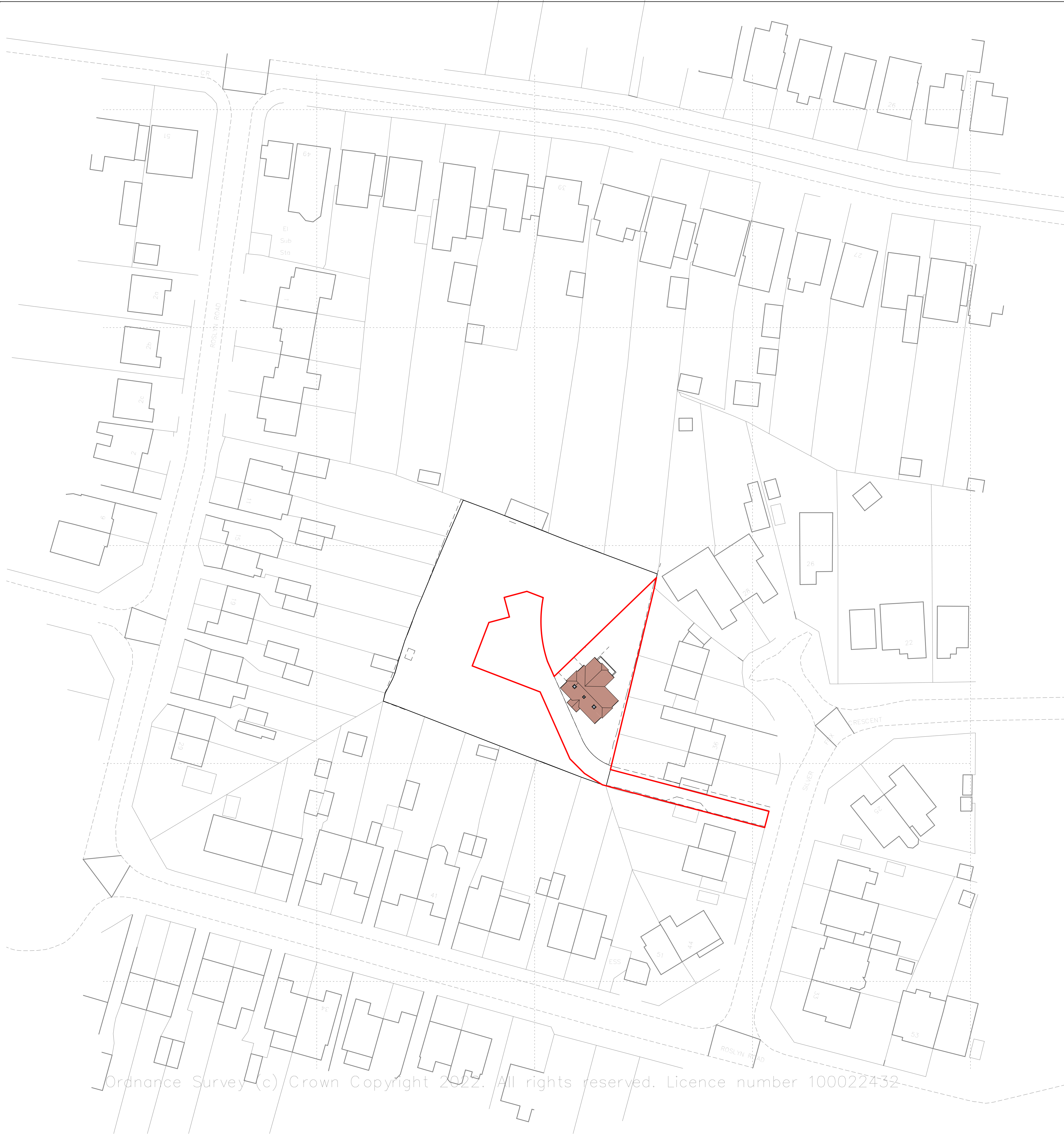
1 Block Plan 1 : 500
