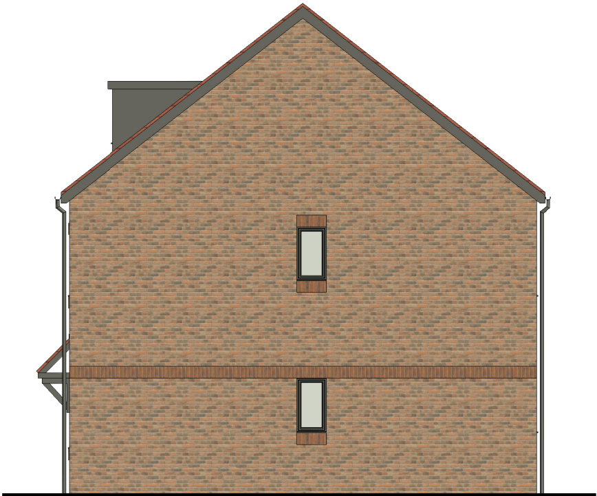
Right Elevation
