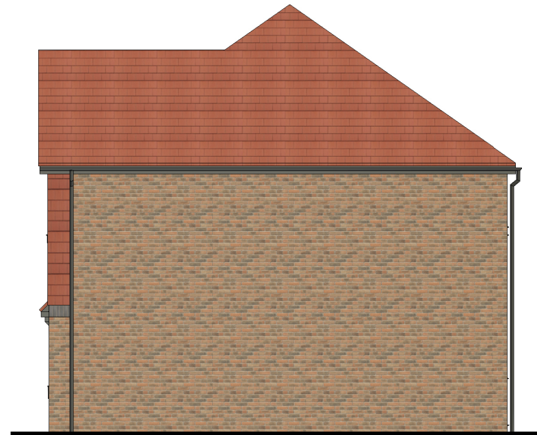
Right Elevation
