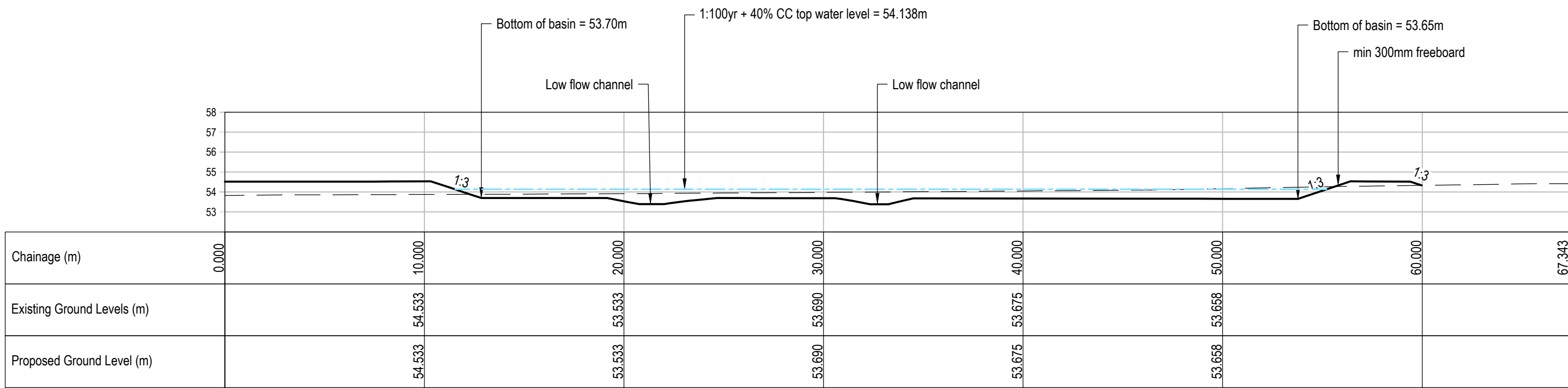
Sports Hub Basin Alignment A-A Scale: H 1:200 V 1:200 Datum 50.000
