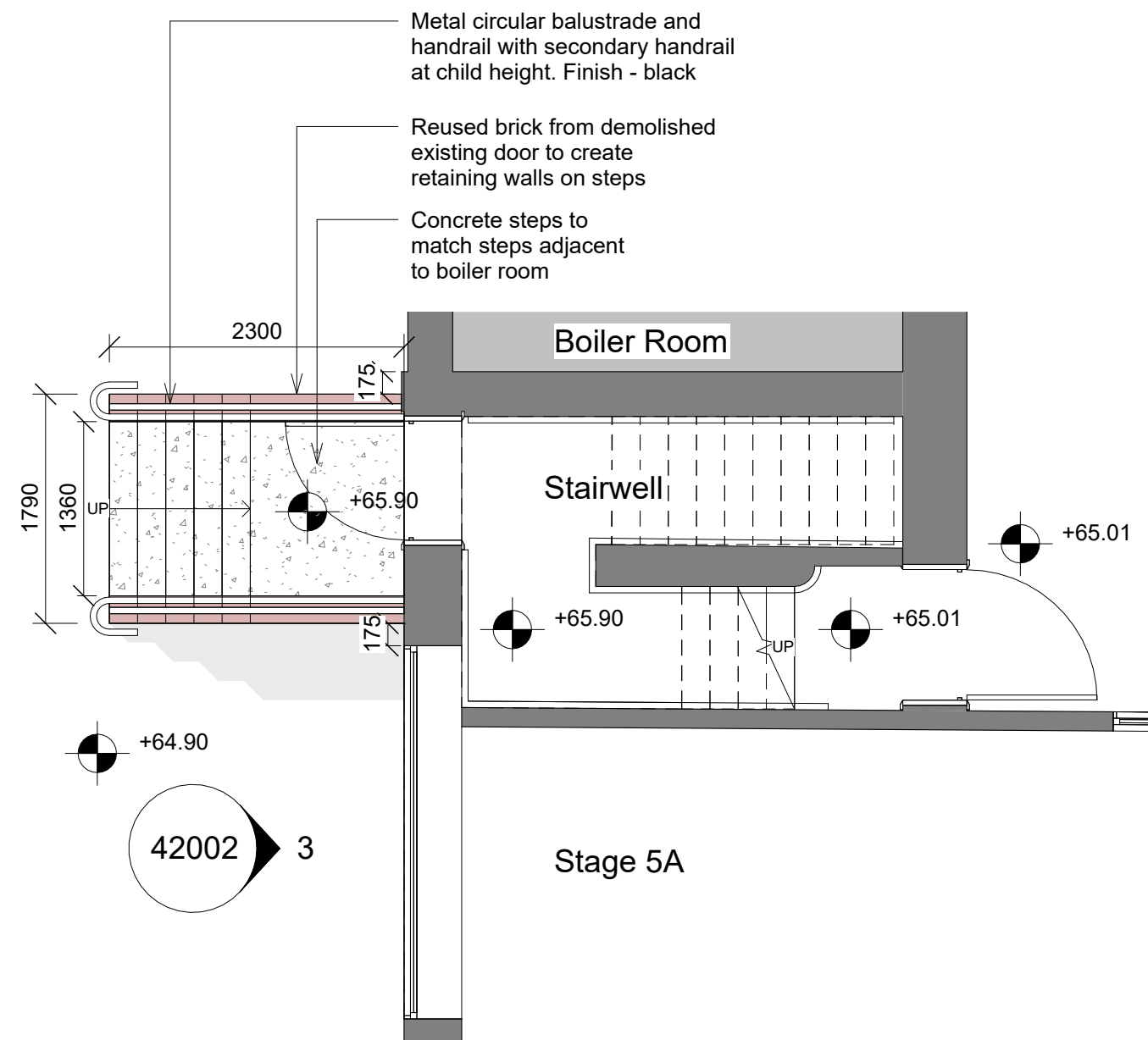
2 00_PLN_KeyPlan_Proposed Fire Door 1 : 50
