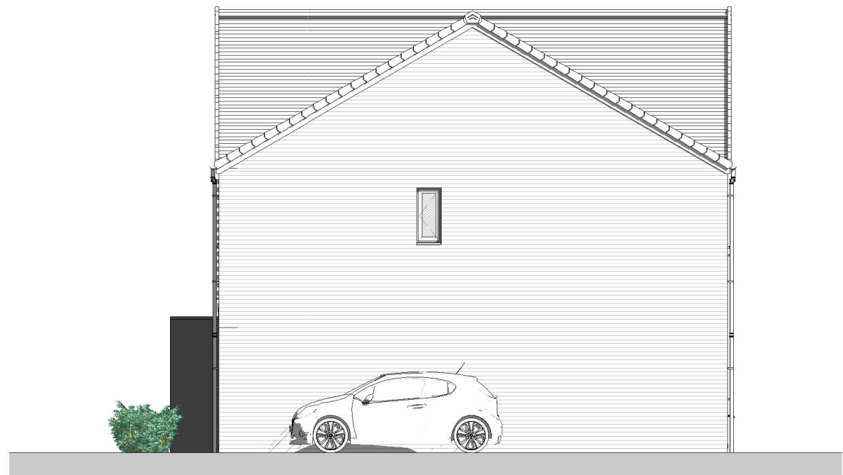
Right Elevation 1 : 100
