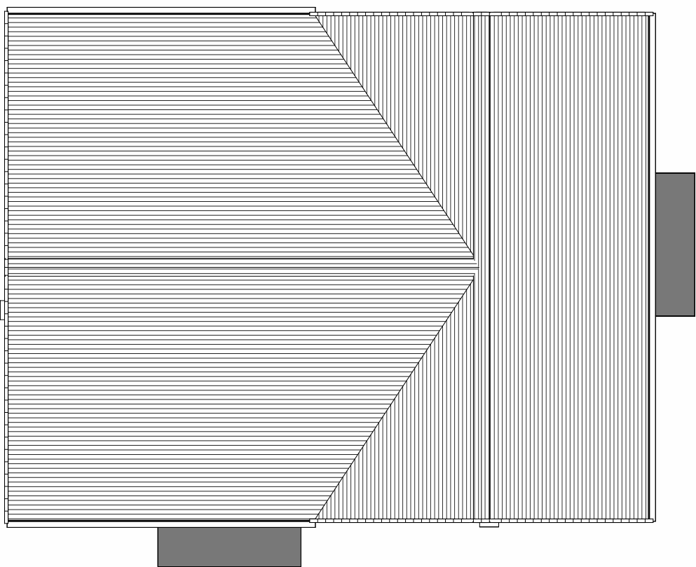
Roof Plan 1 : 100
