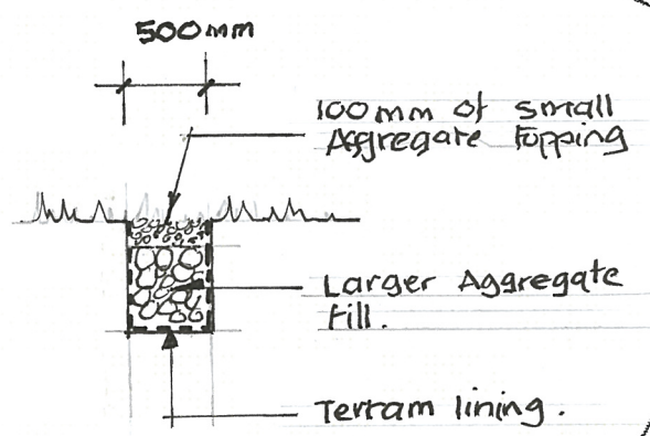
SECTION 1:50 A-A
