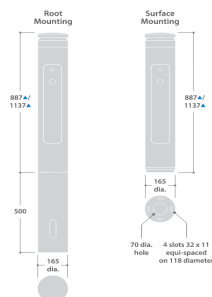
Luminaire Dimension Image
