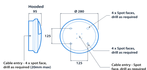
Luminaire Dimension Image
