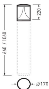
Luminaire Dimension Image
