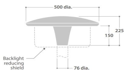
Luminaire Dimension Image
