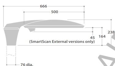
Luminaire Dimension Image
