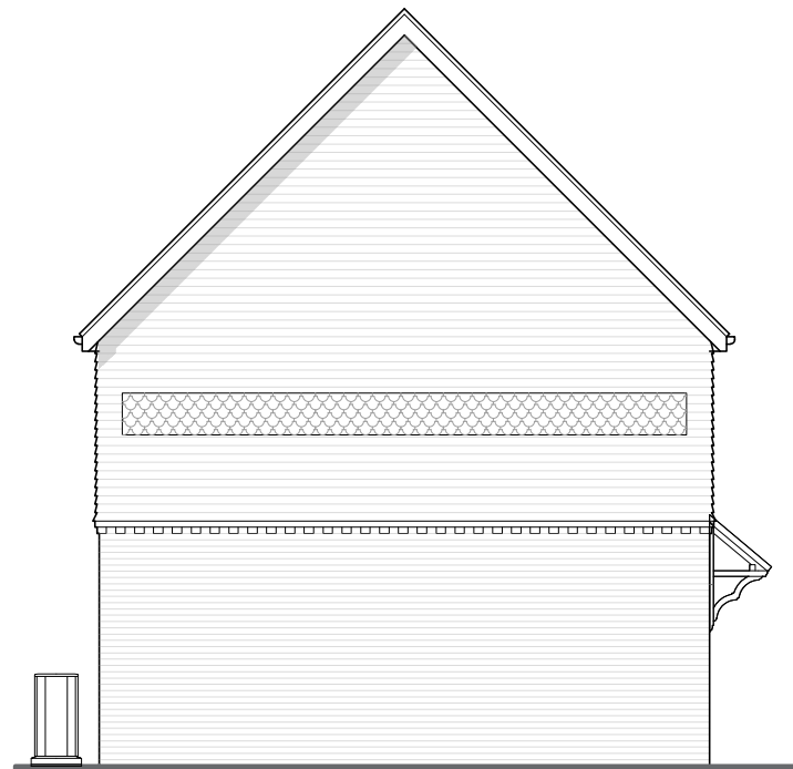
Elevation B
