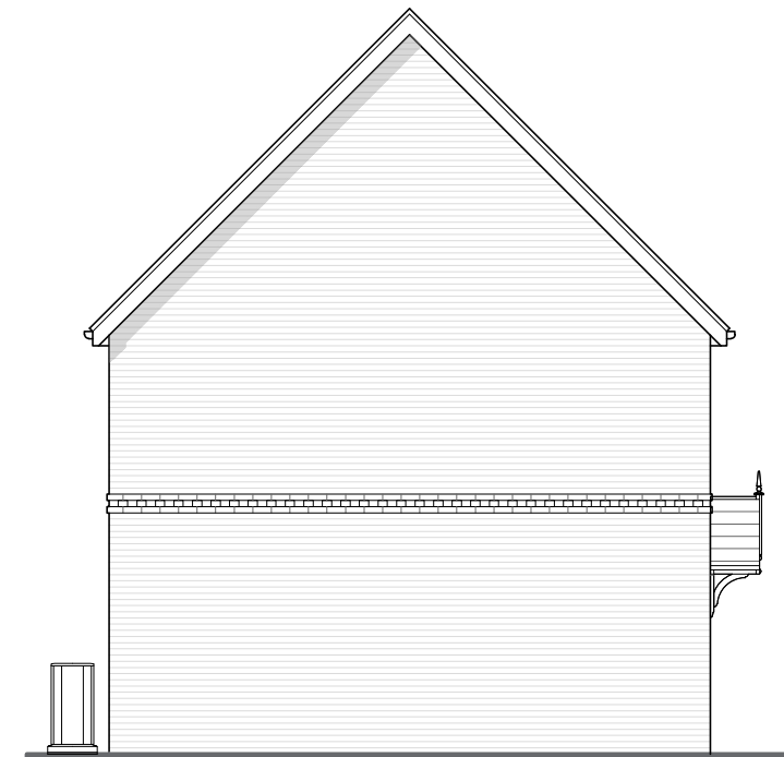
Elevation B
