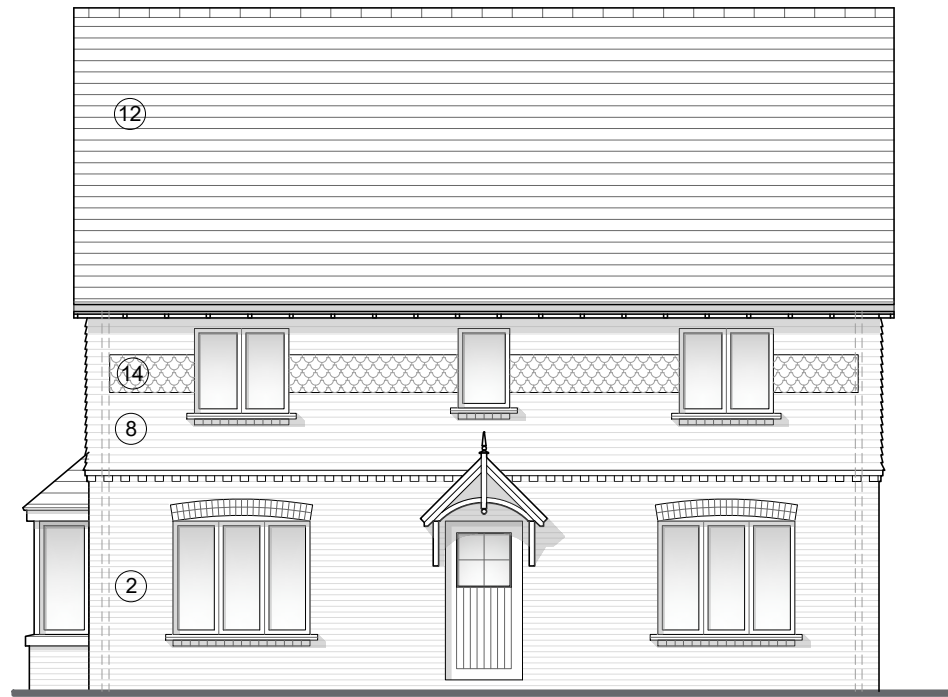
Elevation A
