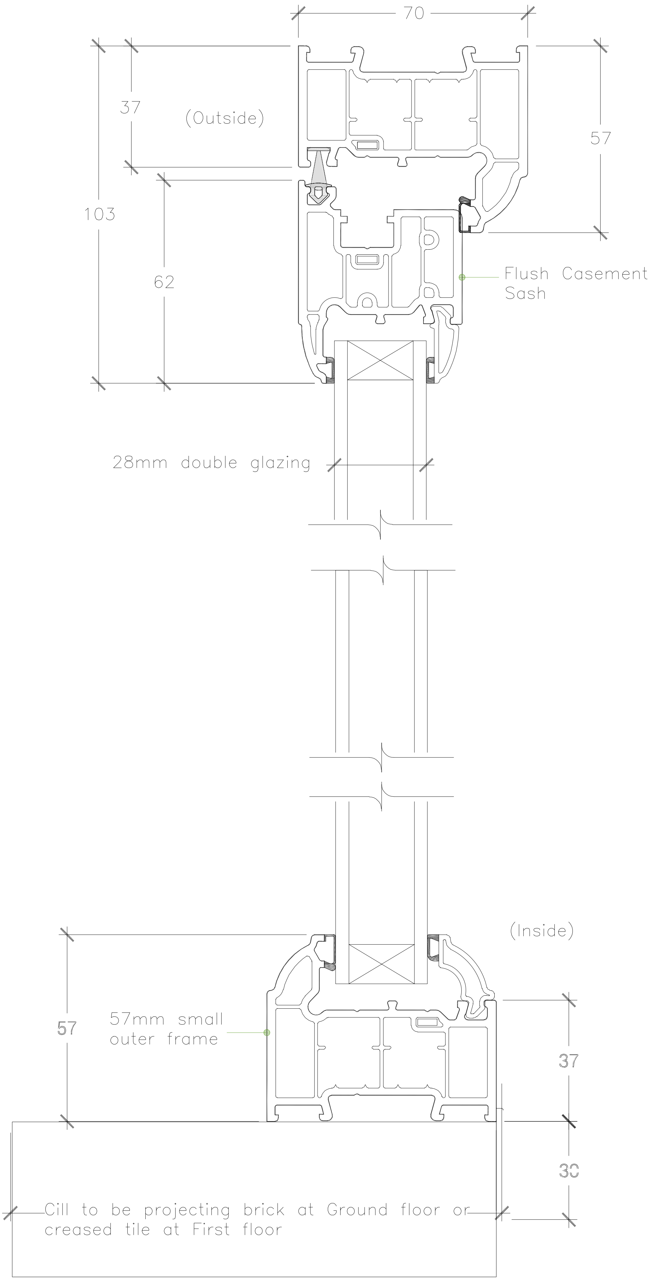
Section A-A
