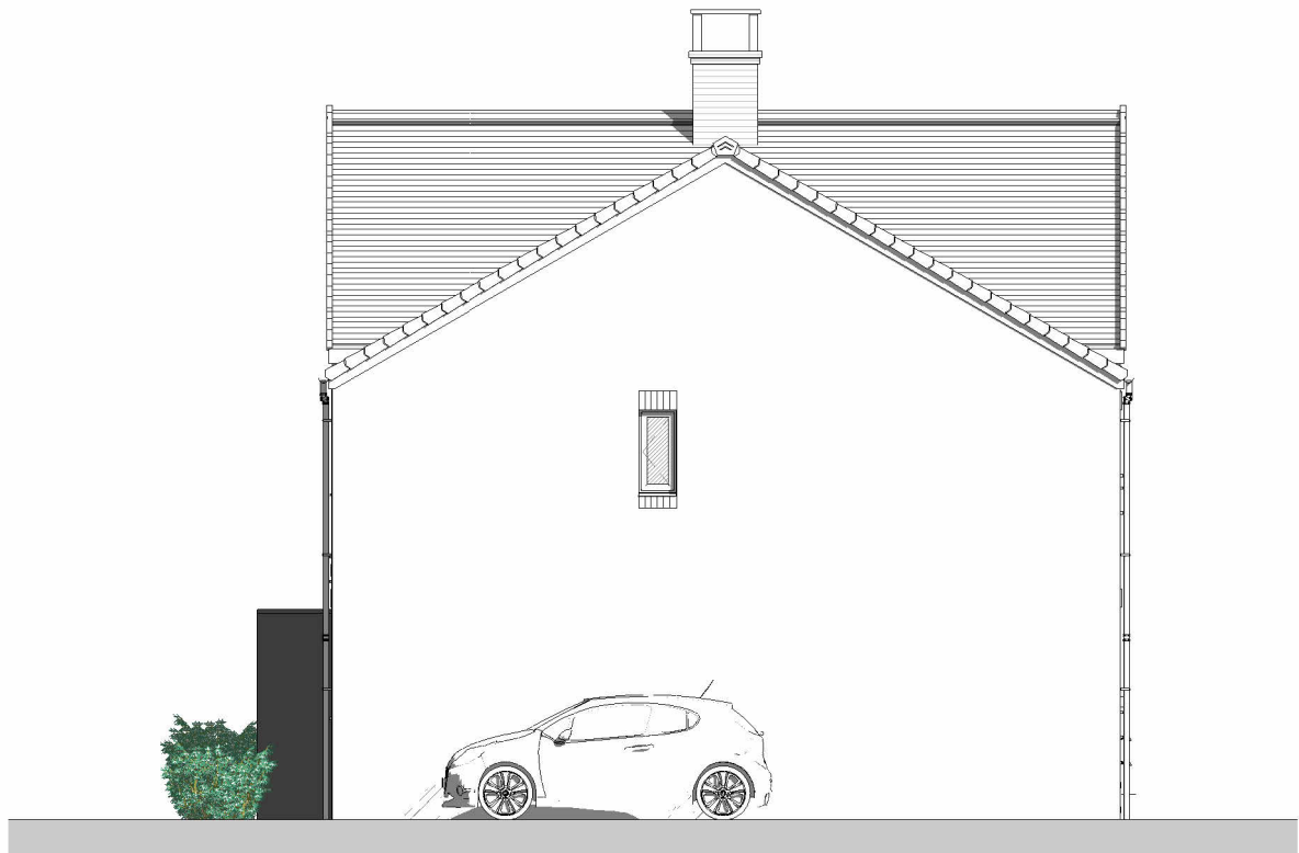
Right Elevation 1 : 100
