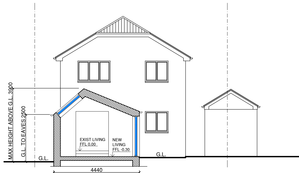
Section A-A 1:100
