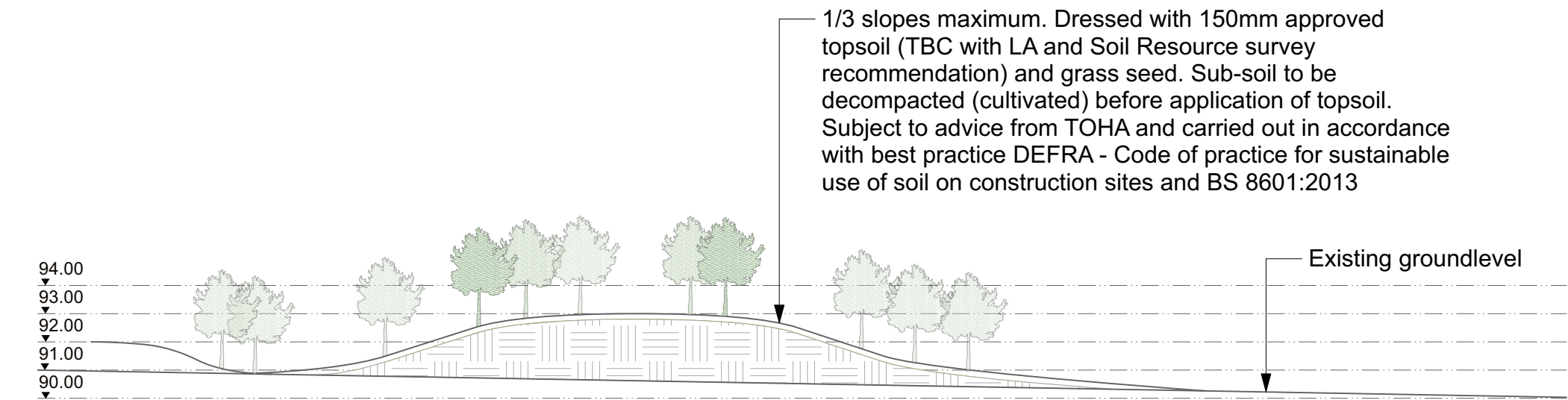
S08 Mound section Scale: 1:200
