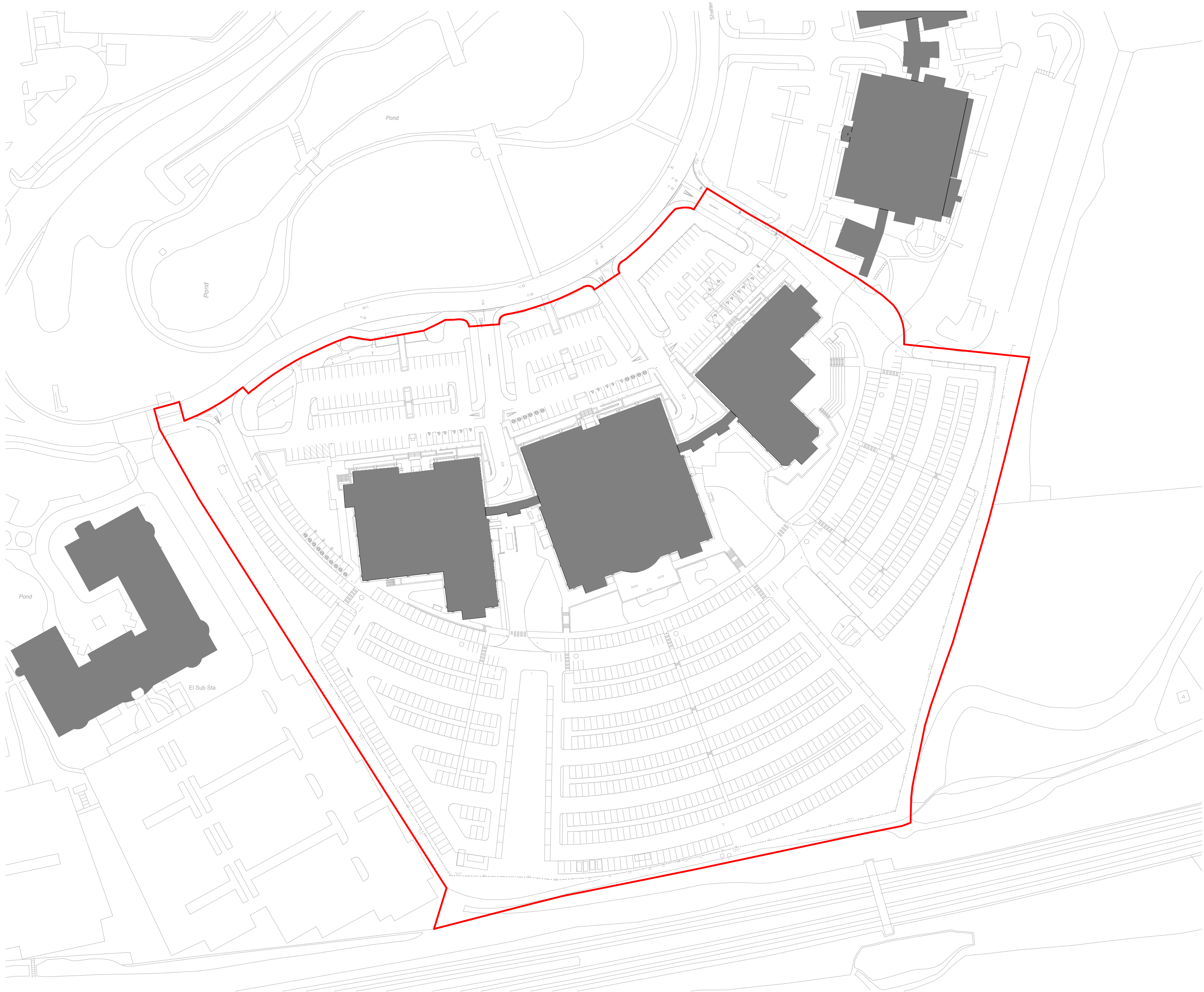
1 Block Plan 1 : 1000
