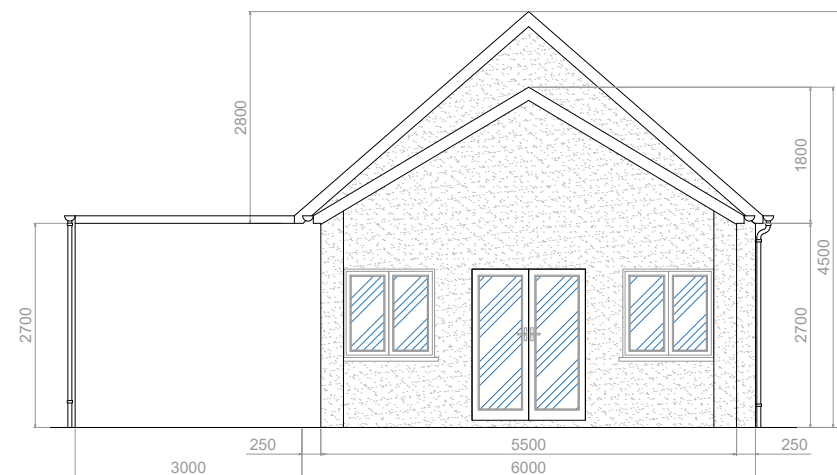
Right Elevation
