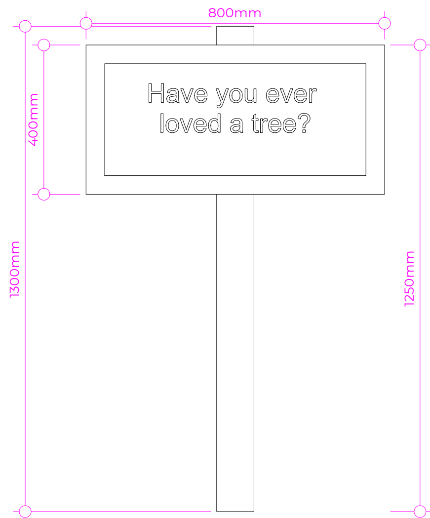
2 FRONT VIEW Scale: 1:10
