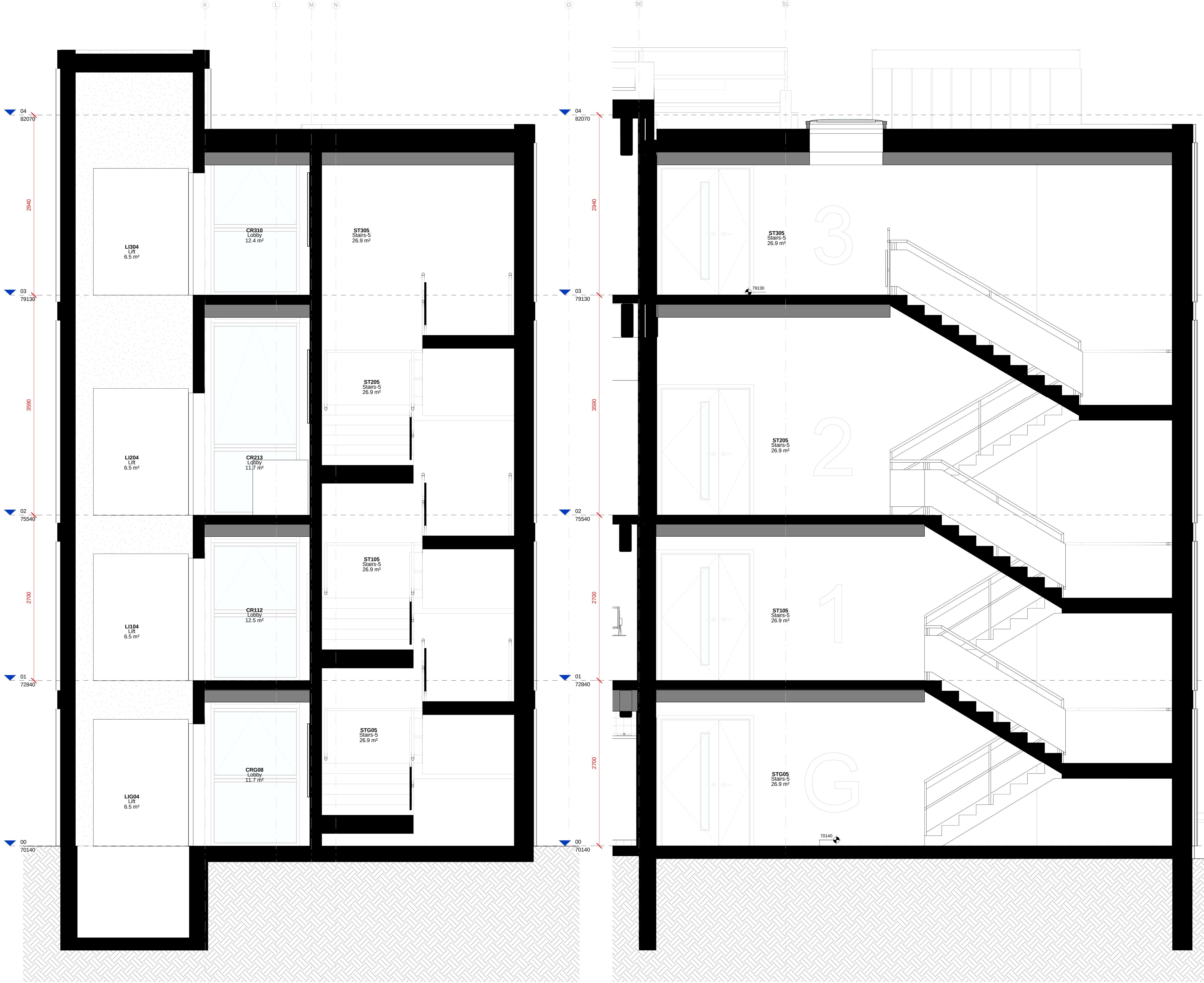
1 | Stair 05 Section 01 1 : 25
