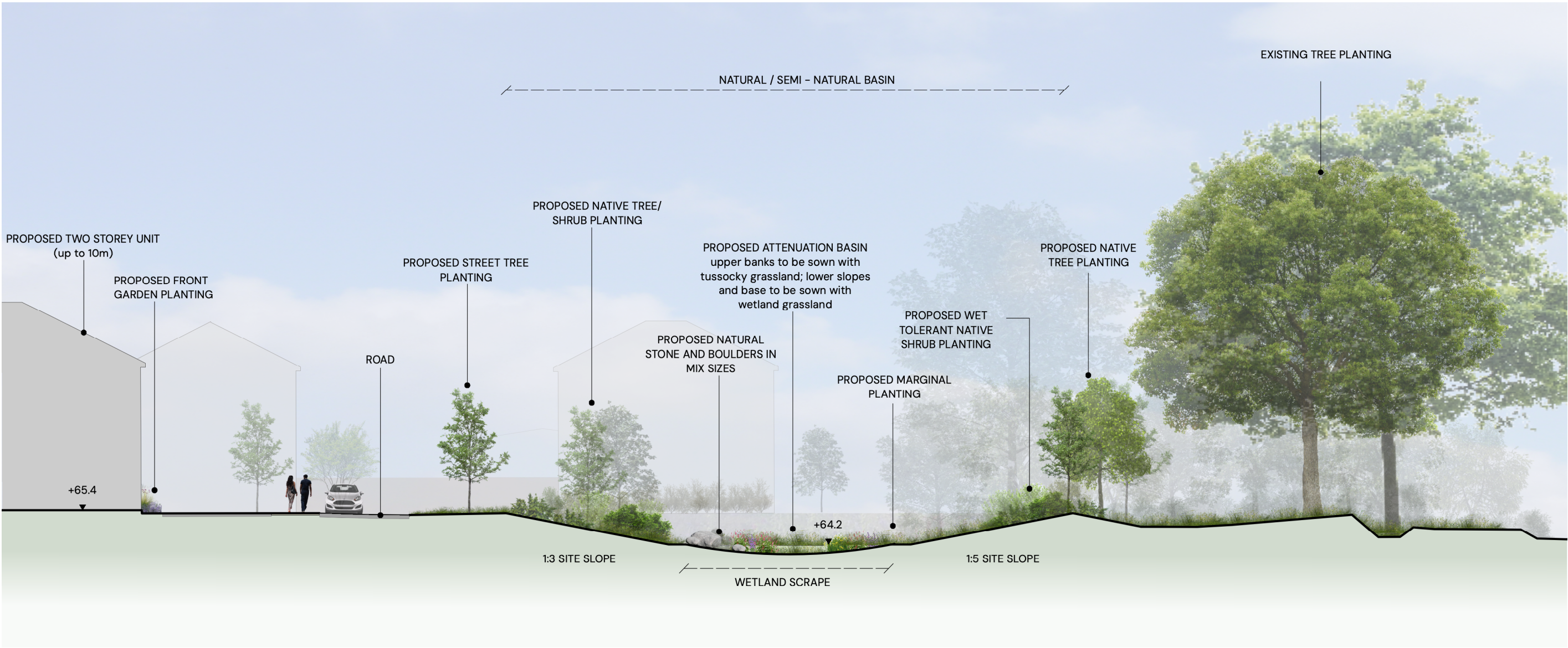
SECTION A-AA
