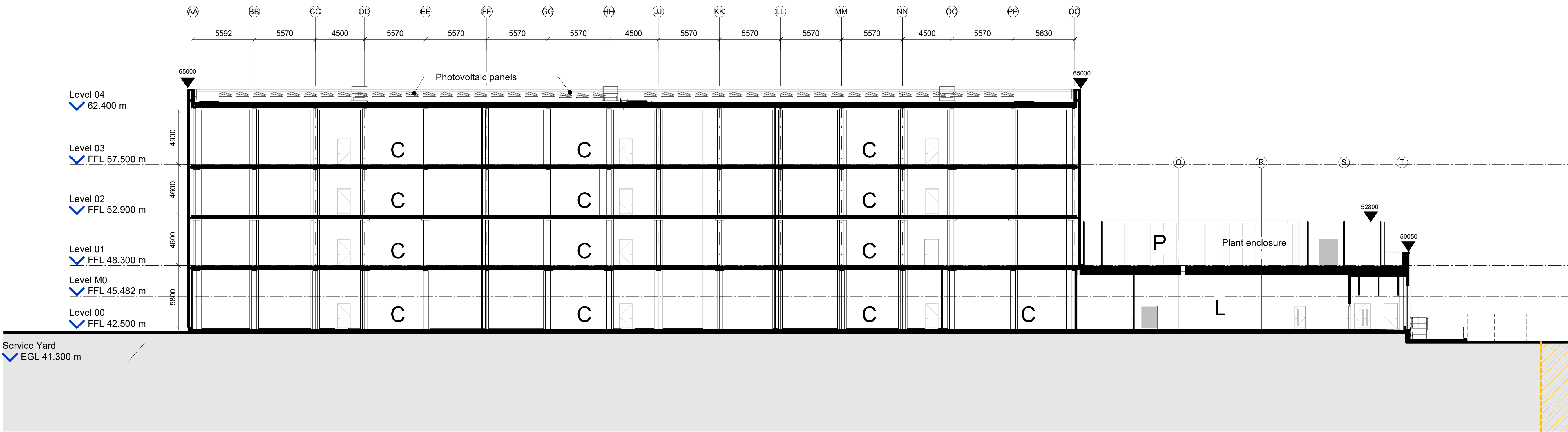
1 Section C-C 1 : 200
