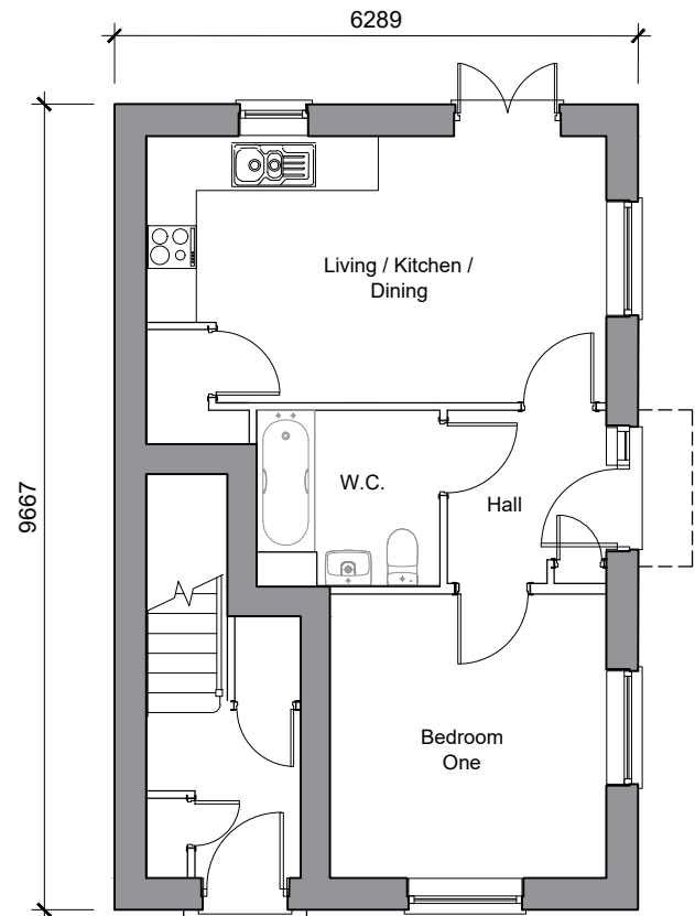
AF1C - 1 Bedroom Maisonette NIA 39.13sqm
