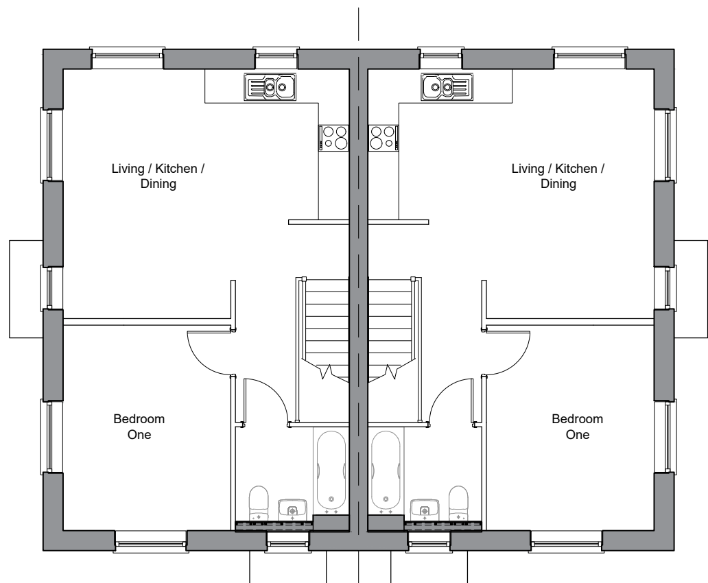
AF1D - 1 Bedroom Maisonette NIA 56.56sqm
