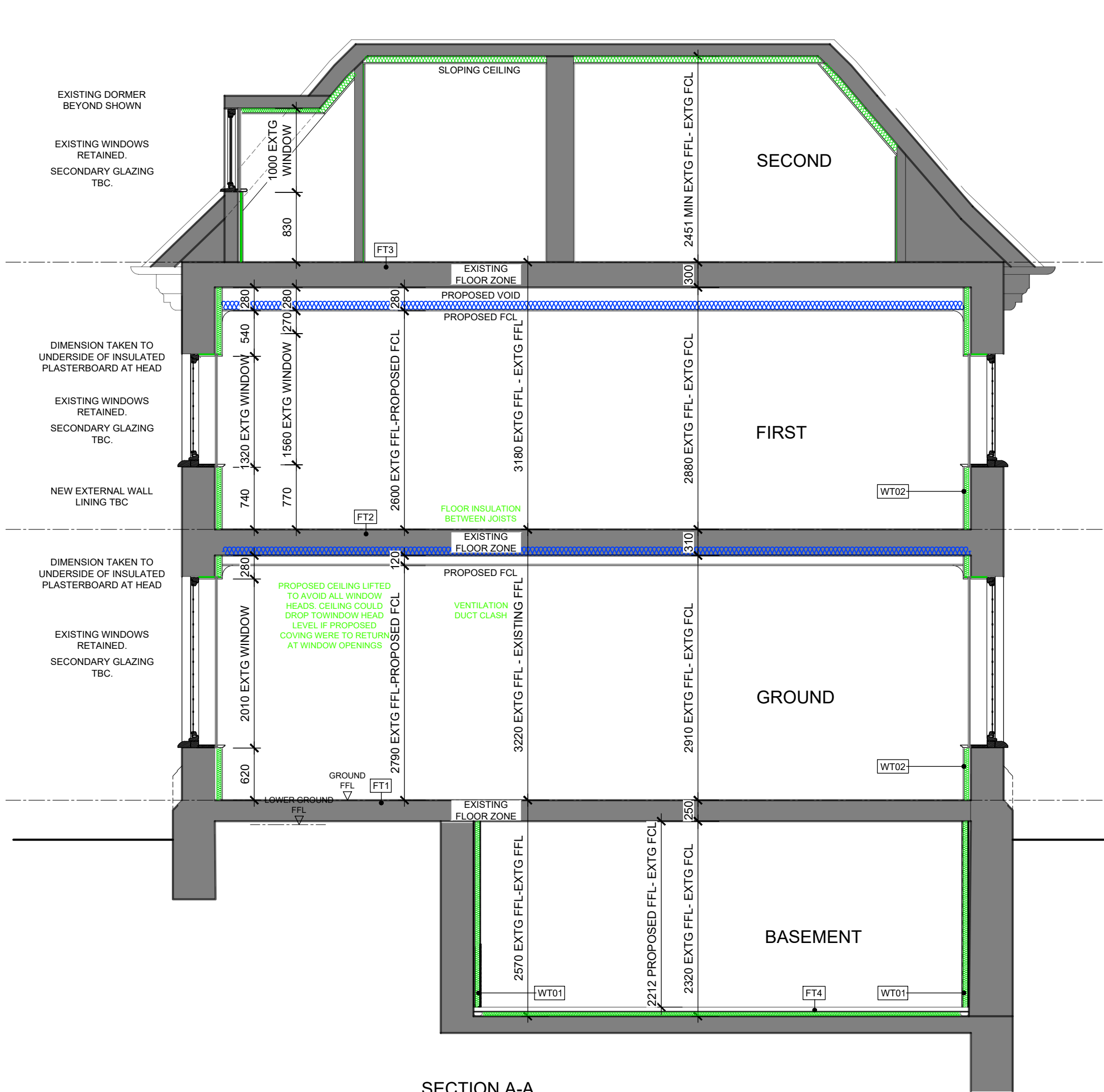
SECTION A-A
