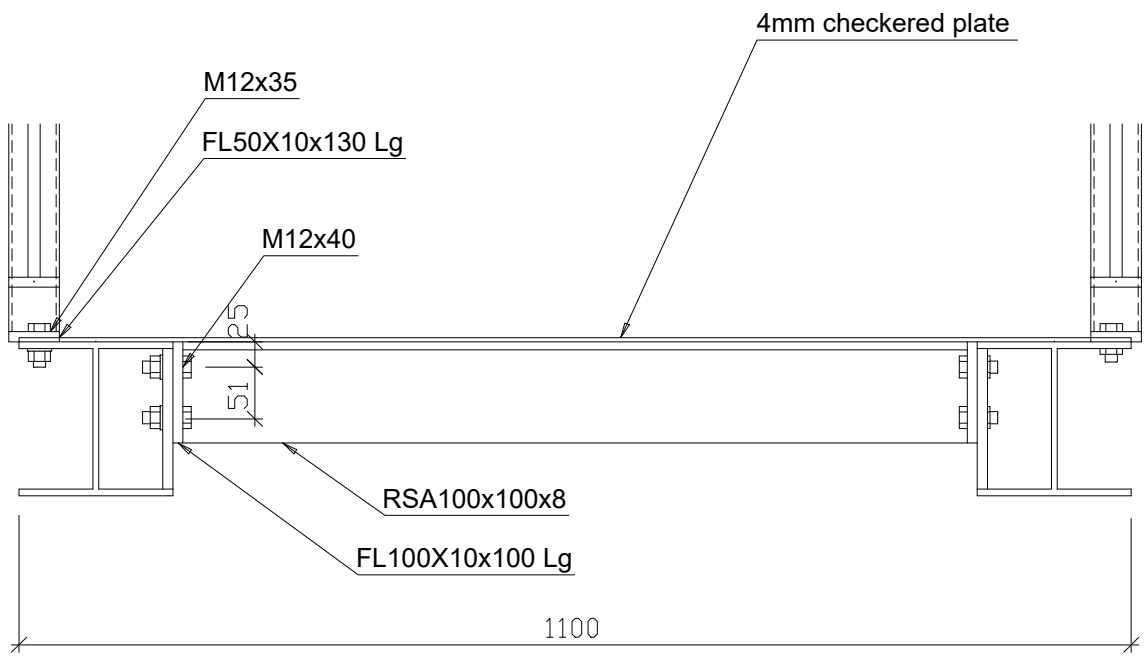
SECTION-A
