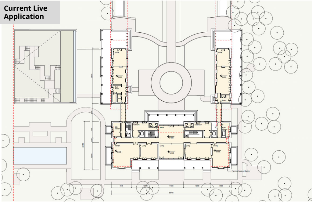
PCY-PBC-MH-00-DR-A-1010 (GF)
