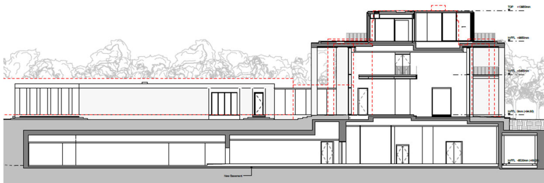
PCY-PBC-MH-ZZ-DR-A-1015 (N/S)
