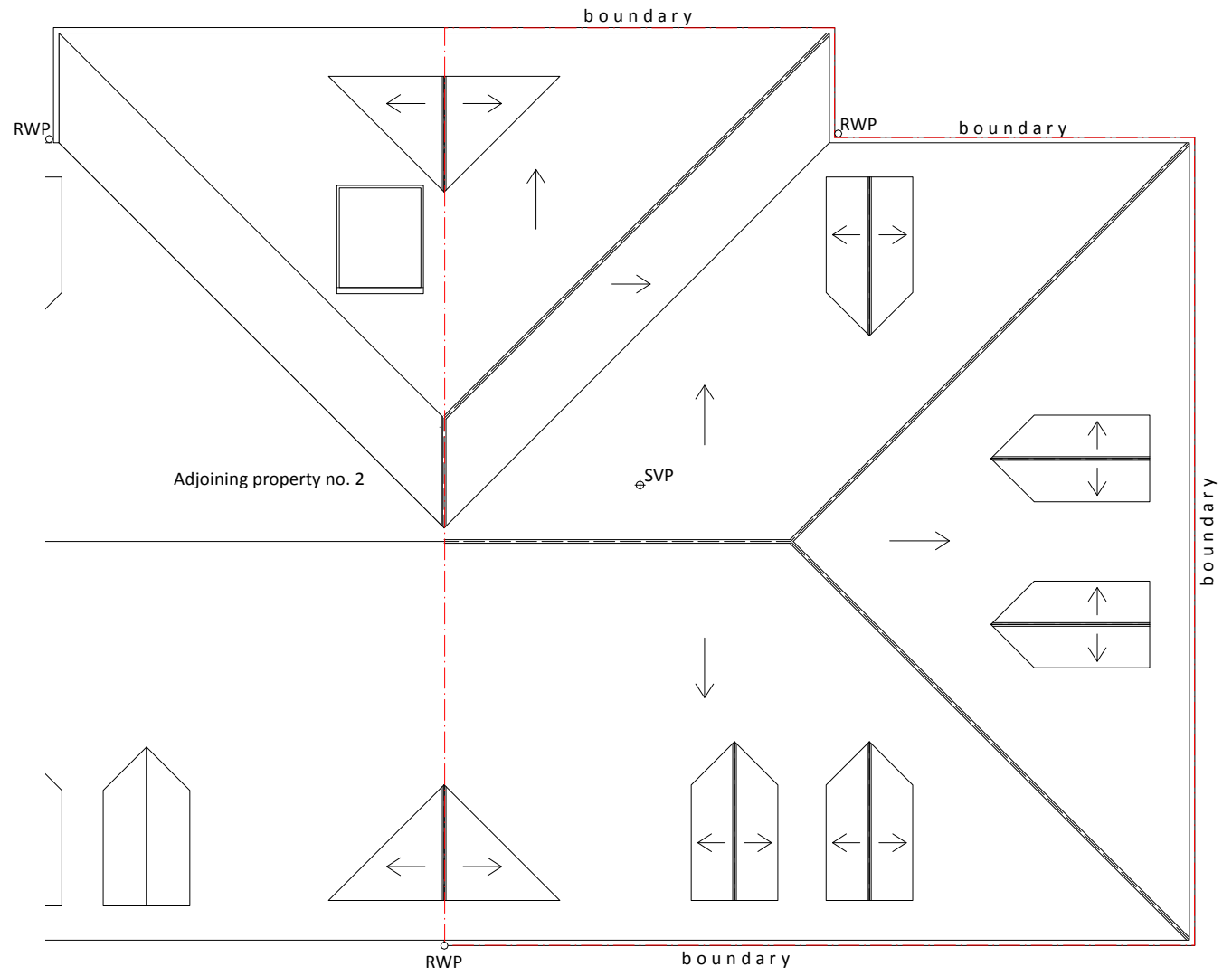
4 ROOF Scale: 1:100
