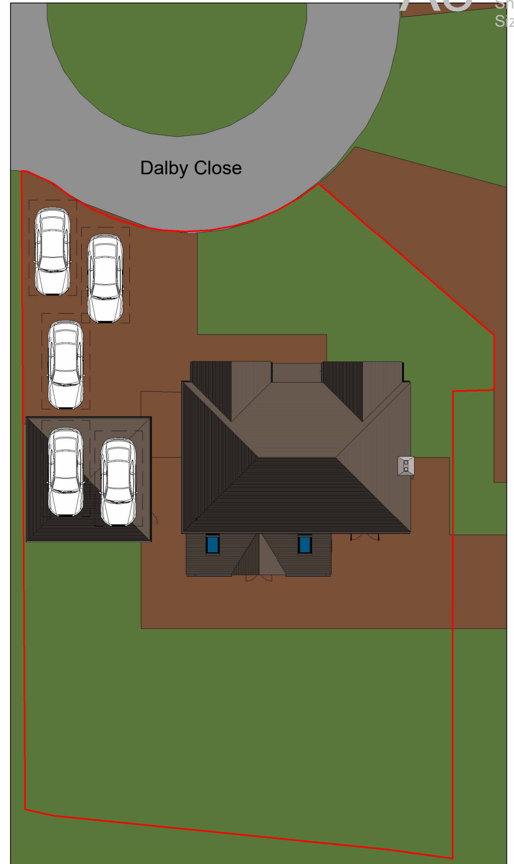
Site Plan Copy 1 1 : 200
