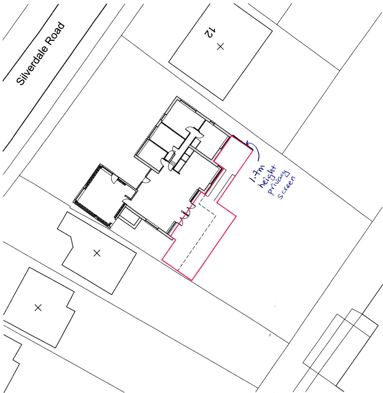
Site Plan 1:200
