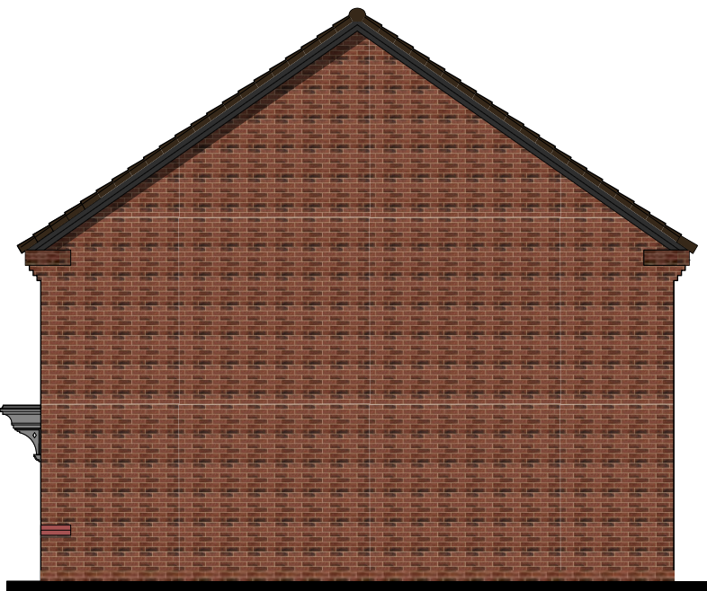
NSS.M3B5P-1 SIDE ELEVATION
