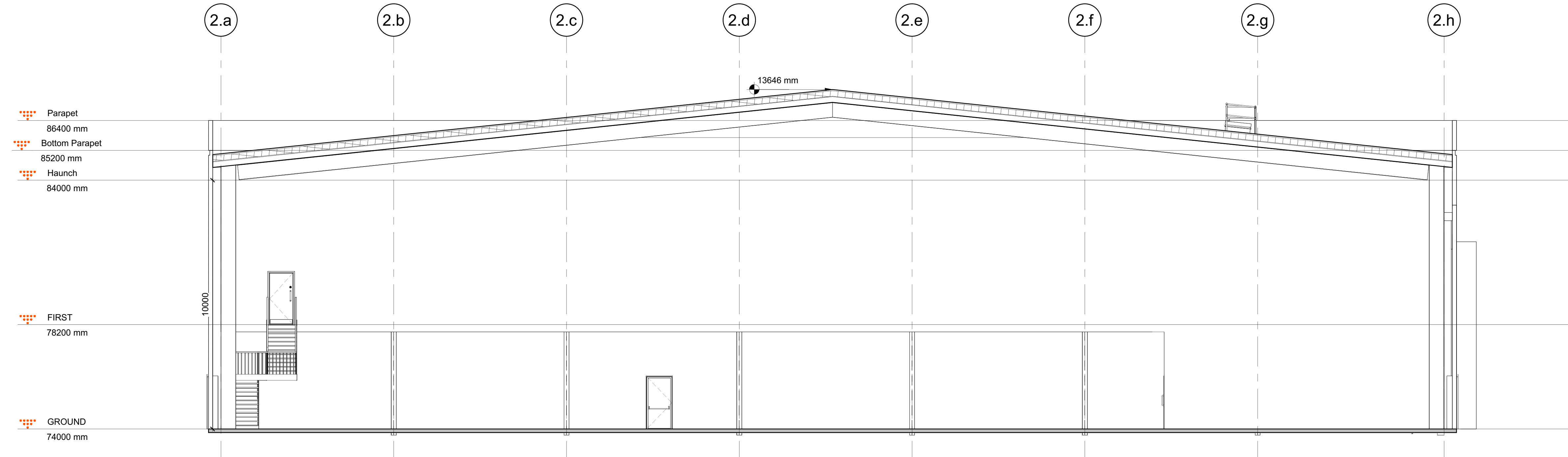
2 Warehouse Section B 1 : 100
