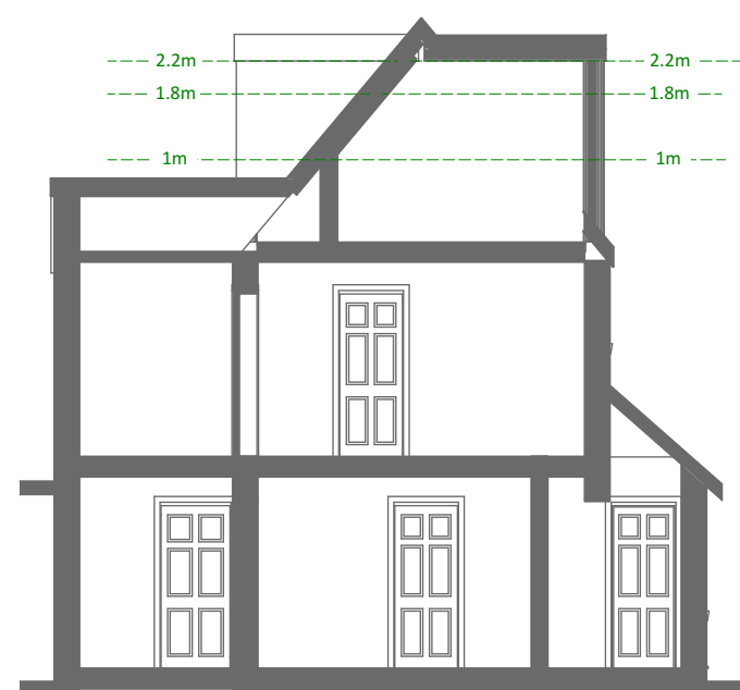
10 Section S-02 1:100
