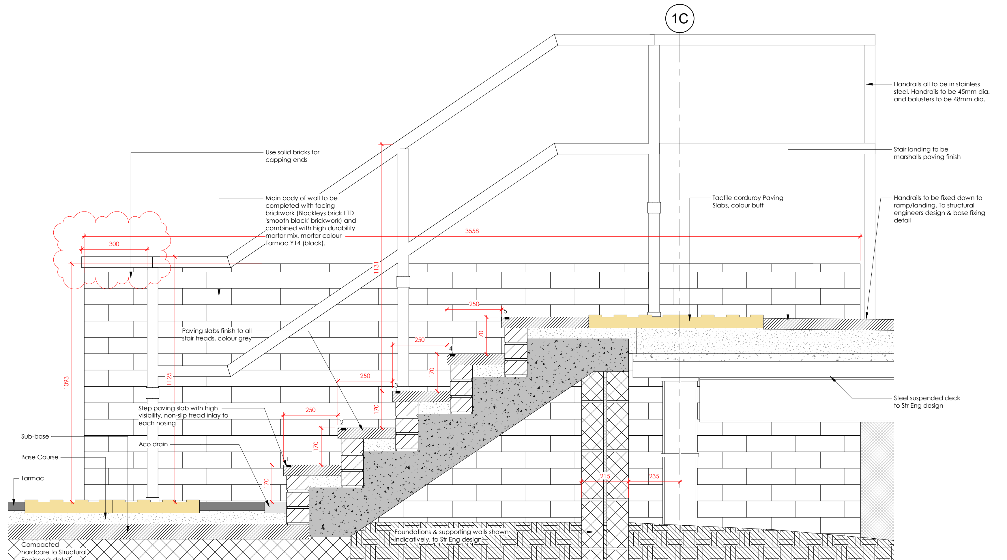
1 STAIR DETAIL 1 : 10
