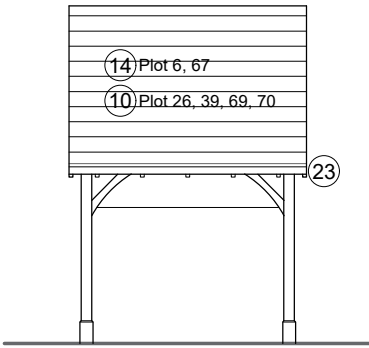
Elevation A
