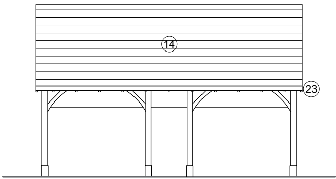
Elevation A
