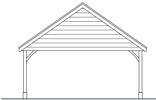
Elevation B
