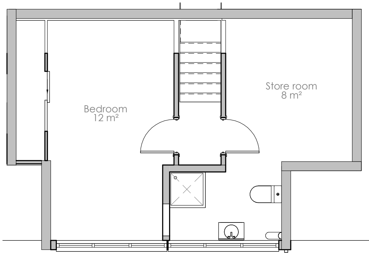
Level 2 - Existing 1 : 50
