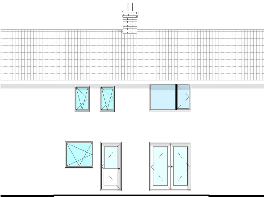
2 Rear 1 : 100
