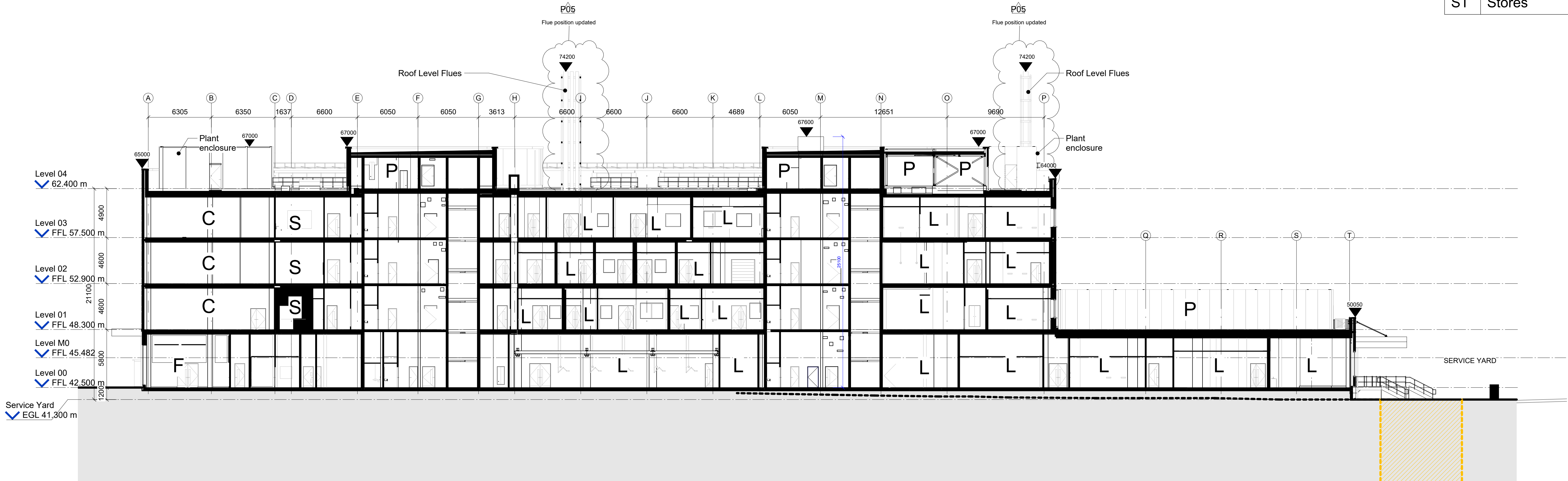
1 Section B-B 1 : 200
