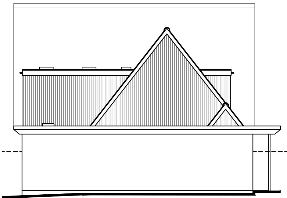
E. Side Elevation 1:100
