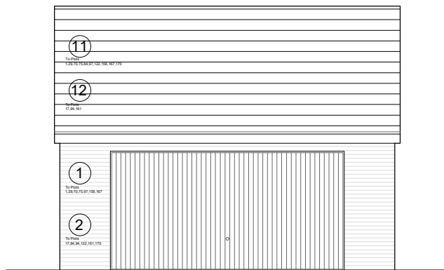
Elevation A
