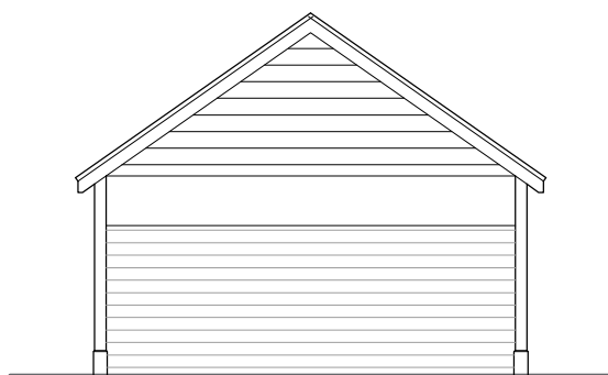
Elevation B
