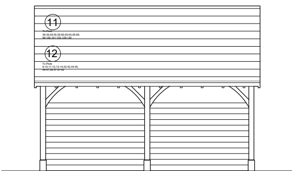
Elevation A
