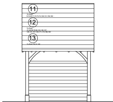
Elevation A
