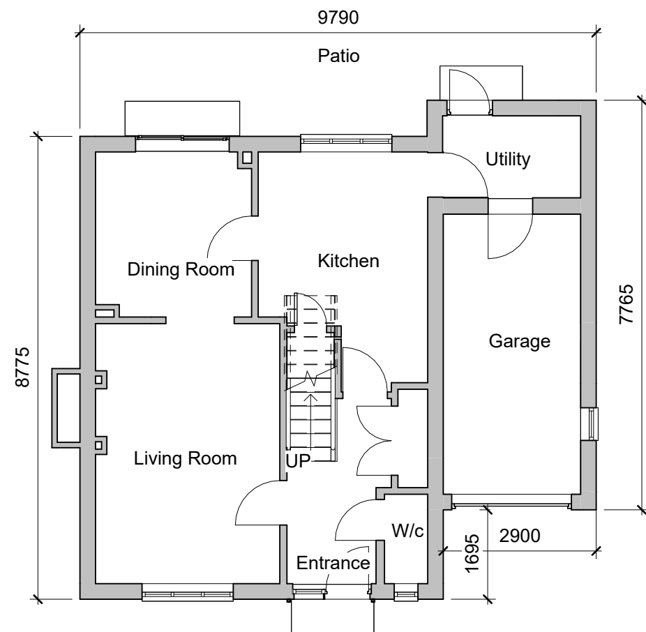
1 Existing GF 1 : 100
