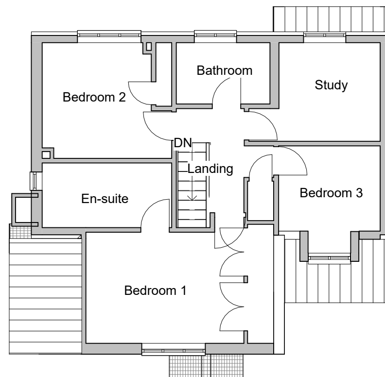
2 Existing FF 1 : 100
