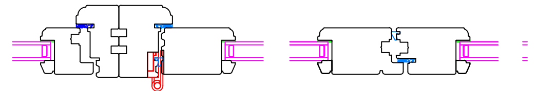
Door Mullion
