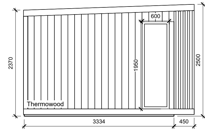
2 LH Elevation 1 : 50
