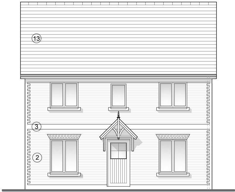
Elevation A
