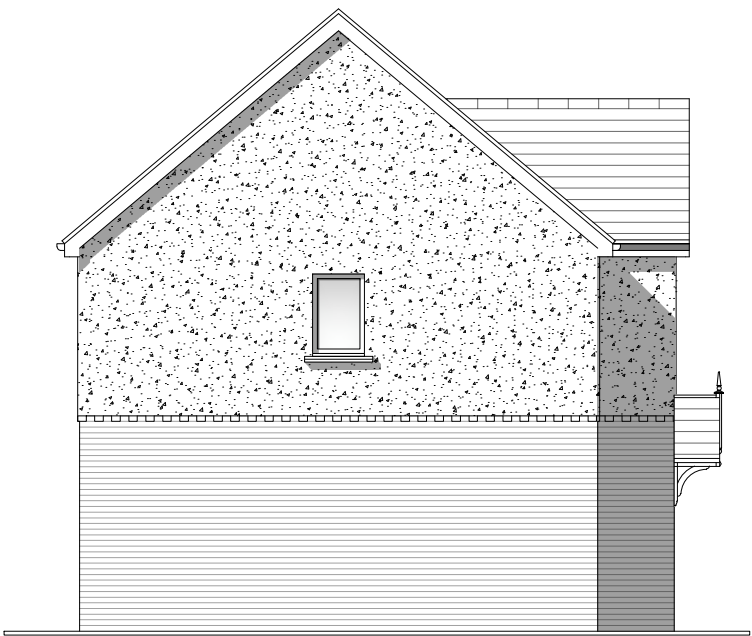
Elevation B
