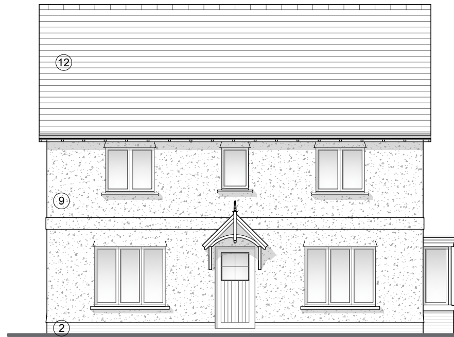
Elevation A
